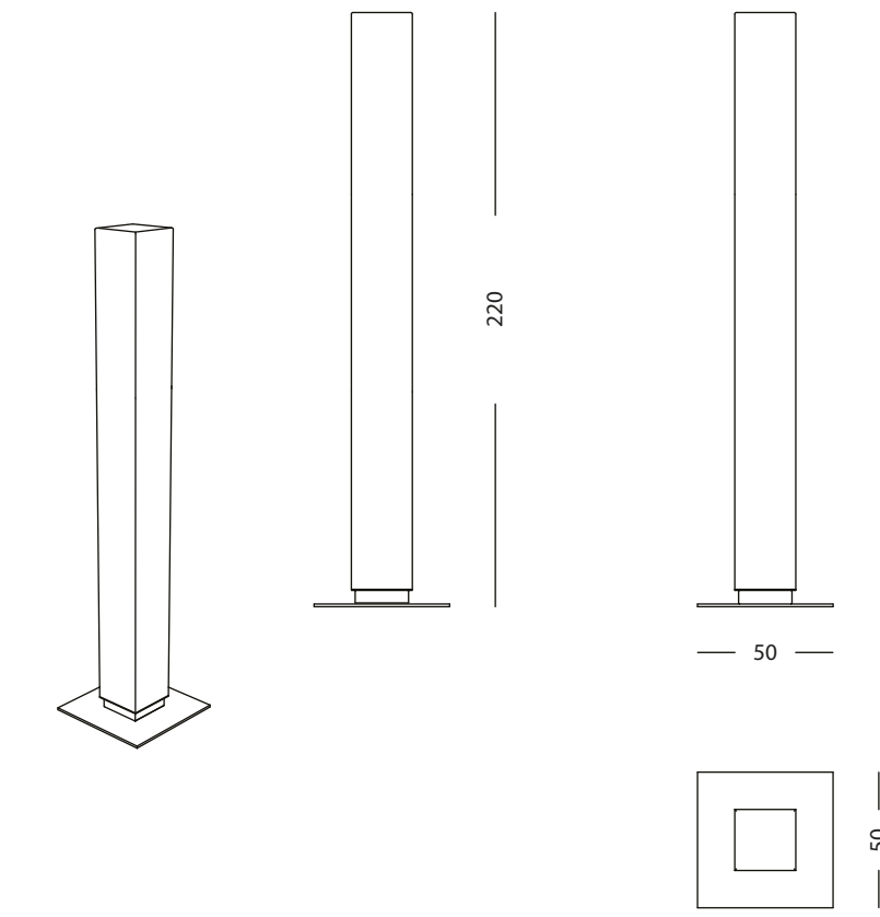
- 16805 Linear lamp 50 x 50 x h 220 cm
