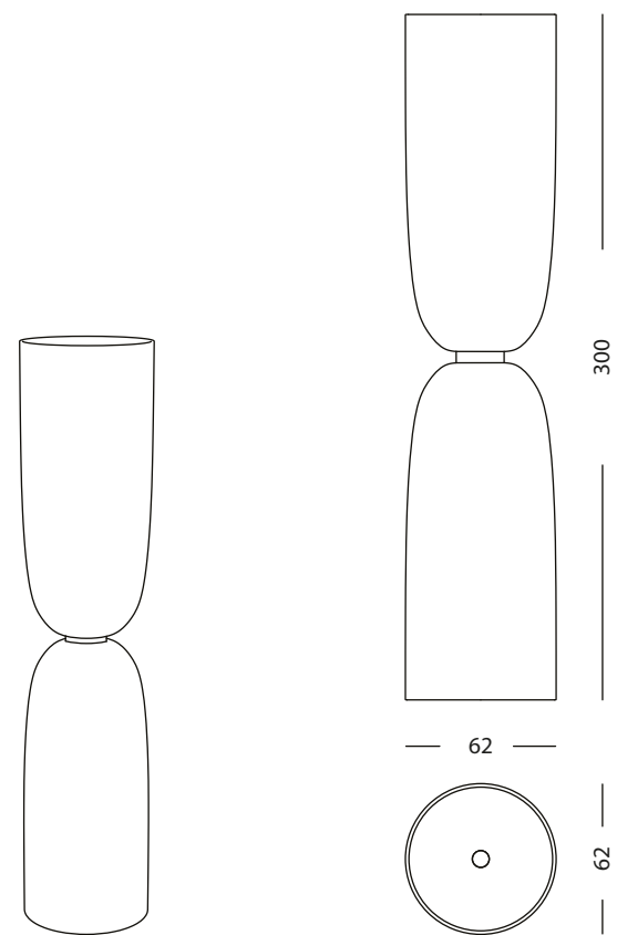
- 66803 Lamp ø 62 x h 300
