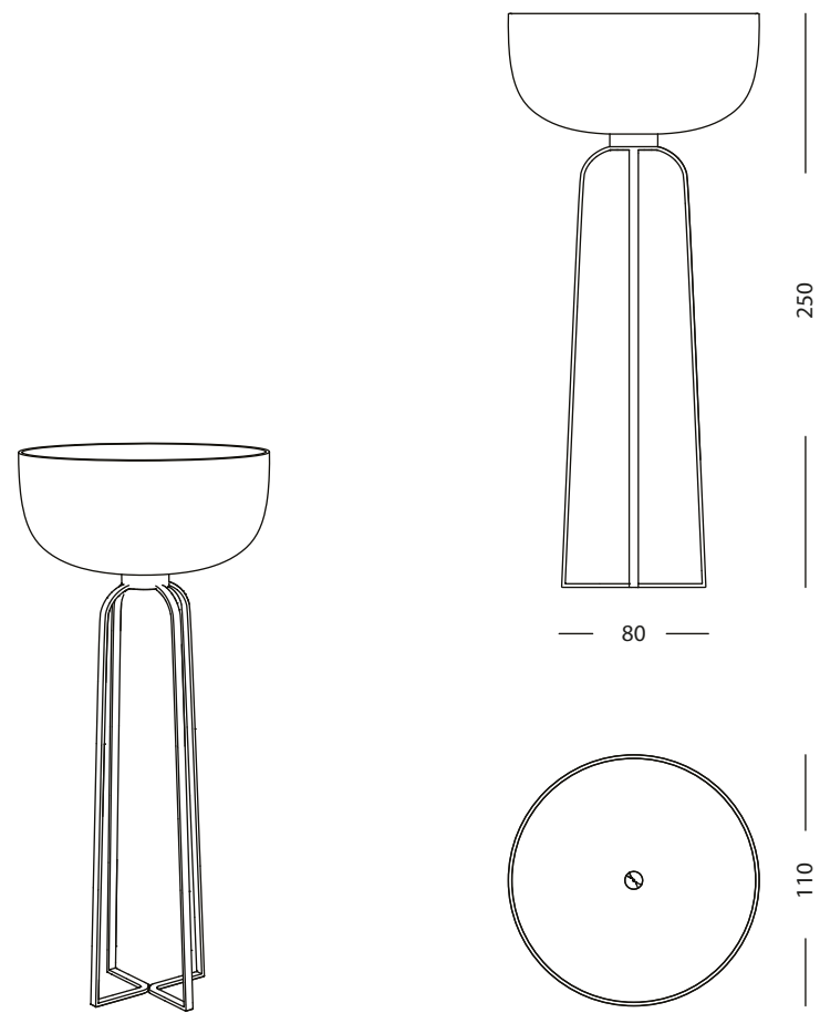
- 66802 Lamp ø 110 x h 250
